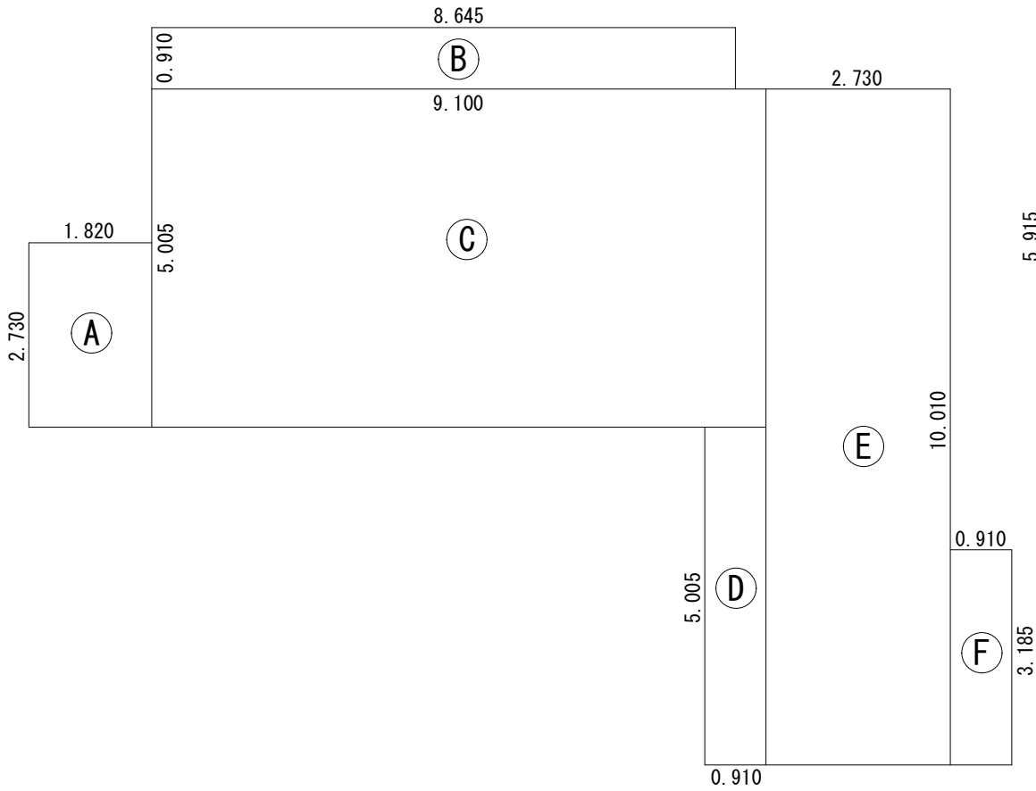
建築面積求積図 S=1/100
